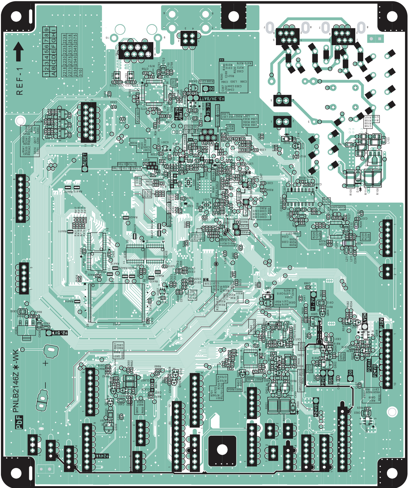
KX-MB2230EU / KX-MB2270EU / KX-MB2515EU / KX-MB2545EU / KX-MB2575EU / DP-MB310EU MAIN BOARD BOTTOM VIEW
