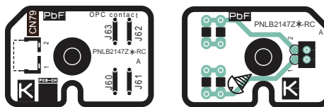
KX-MB2230EU / KX-MB2270EU / KX-MB2515EU / KX-MB2545EU / KX-MB2575EU / DP-MB310EU OPC CONTACT BOARD
