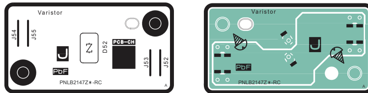
KX-MB2230EU / KX-MB2270EU / KX-MB2515EU / KX-MB2545EU / KX-MB2575EU / DP-MB310EU VARISTOR BOARD
