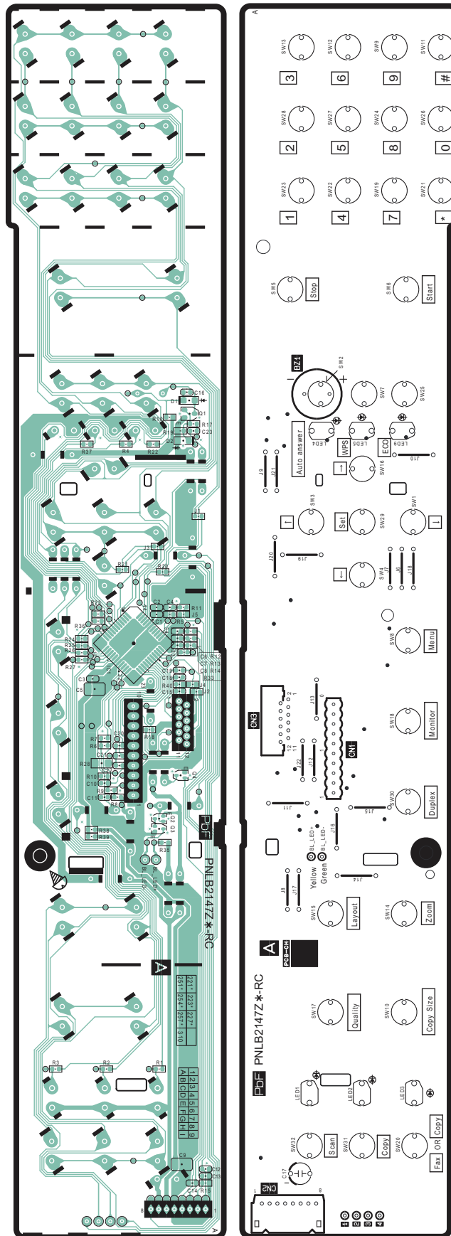
KX-MB2230EU / KX-MB2270EU / KX-MB2515EU / KX-MB2545EU / KX-MB2575EU / DP-MB310EU OPERATION PANEL BOARD
