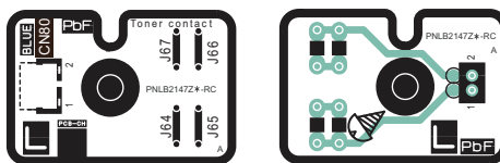
KX-MB2230EU / KX-MB2270EU / KX-MB2515EU / KX-MB2545EU / KX-MB2575EU / DP-MB310EU TONER CONTACT BOARD
