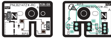
KX-MB2230EU / KX-MB2270EU / KX-MB2515EU / KX-MB2545EU / KX-MB2575EU / DP-MB310EU RPS BOARD
