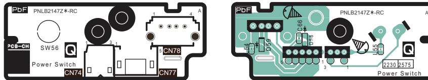
KX-MB2230EU / KX-MB2270EU / KX-MB2515EU / KX-MB2545EU / KX-MB2575EU / DP-MB310EU POWER SWITCH BOARD
