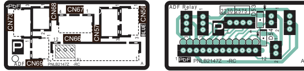
KX-MB2230EU / KX-MB2270EU / KX-MB2515EU / KX-MB2545EU / KX-MB2575EU / DP-MB310EU ADF RELAY BOARD
