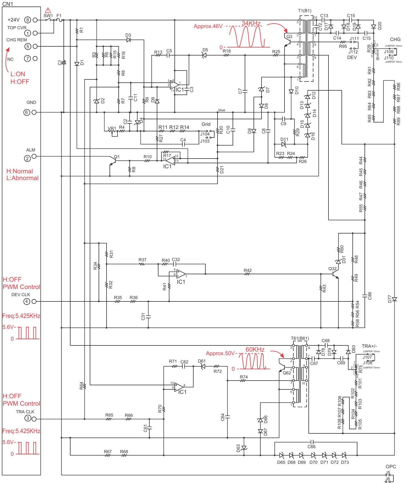
KX-MB2230EU / KX-MB2270EU / KX-MB2515EU / KX-MB2545EU / KX-MB2575EU / DP-MB310EU HIGH VOLTAGE POWER SUPPLY BOARD
