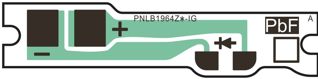
KX-MB2515EU / KX-MB2545EU / KX-MB2575EU / DP-MB310EU Back Light BOARD
